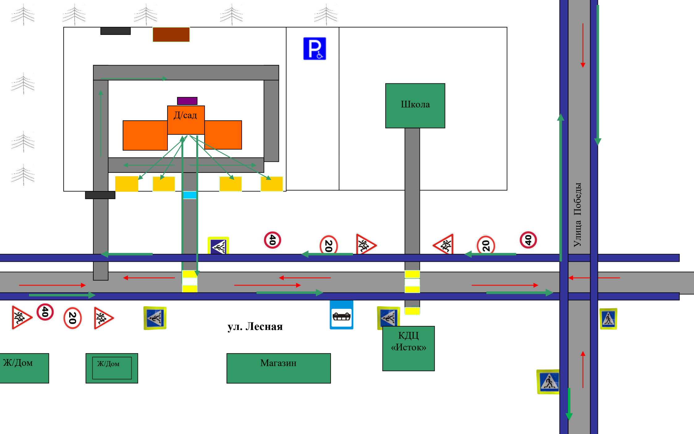
Схема 1 Район расположения МБДОУ, пути движения транспортных средств и детей
