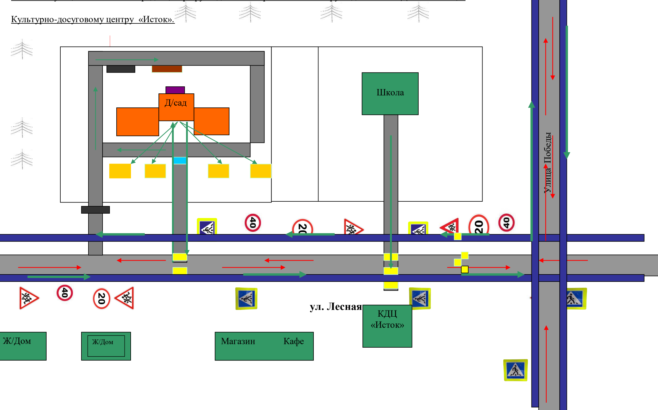
Схема 2 Организация дорожного движения в непосредственной близости от образовательного учреждения с размещением соответствующих технических средств, маршруты движения организованных групп детей от МБДОУ к школе, к
